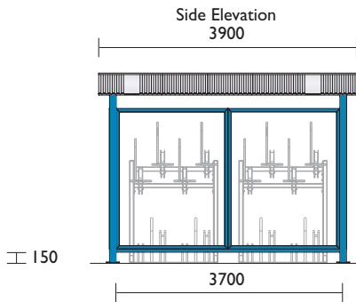
50 x 10mm timber slats INFILLTIM50
